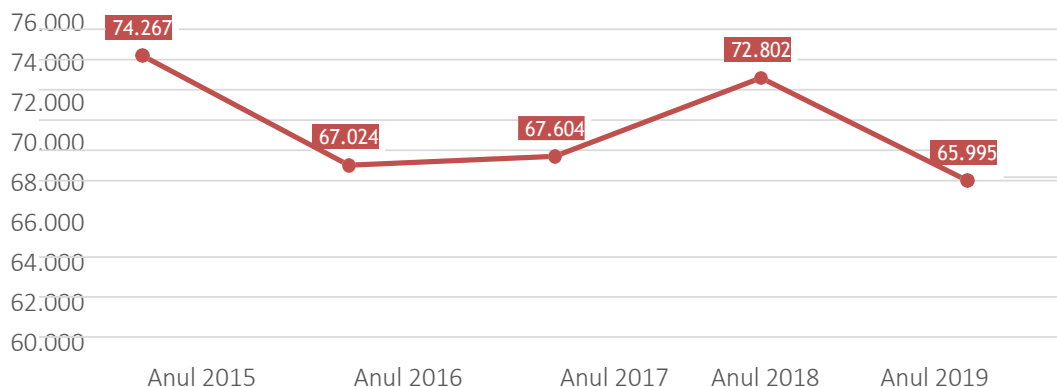
Figura 6-1 - Cantitate energie termică la nivel județean, gigacalorii în perioada 2015-2019 189
