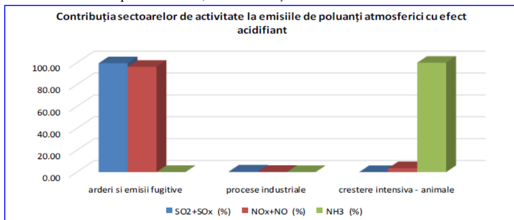
Figura nr. 2. Contribuția sectoarelor de activitate la emisiile de poluanți acidifișanți
